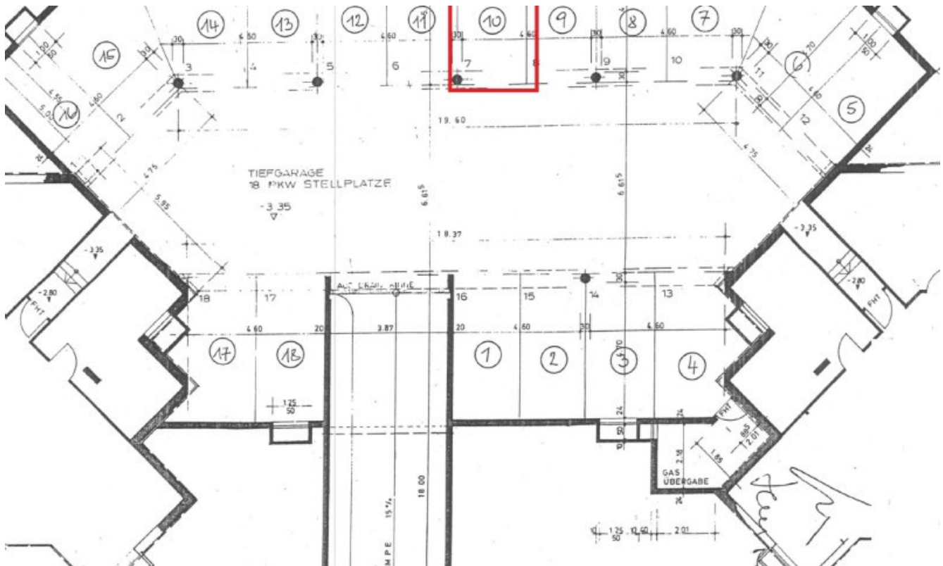
TG (Grundriss)
