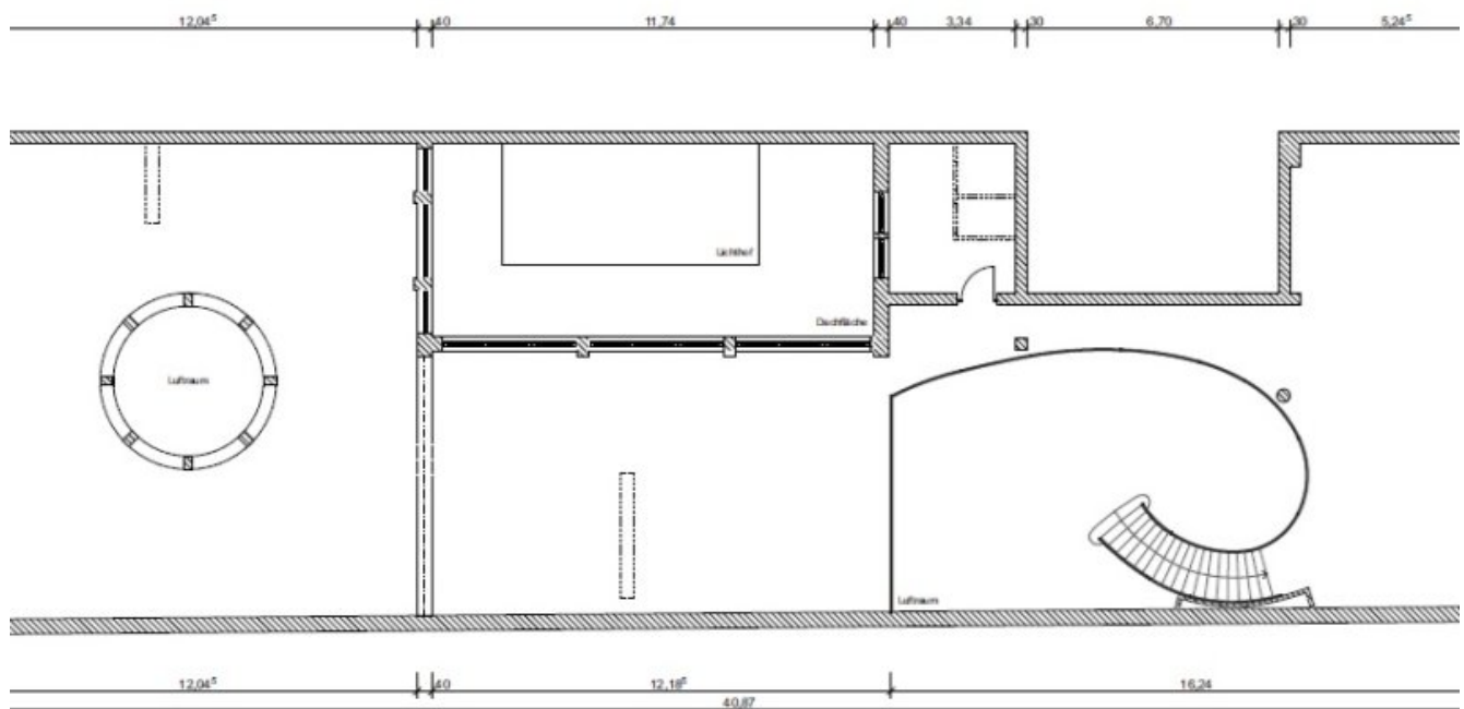
GrundrissplanZGneu (Grundriss)
