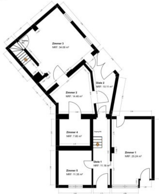
Erdgeschoss
