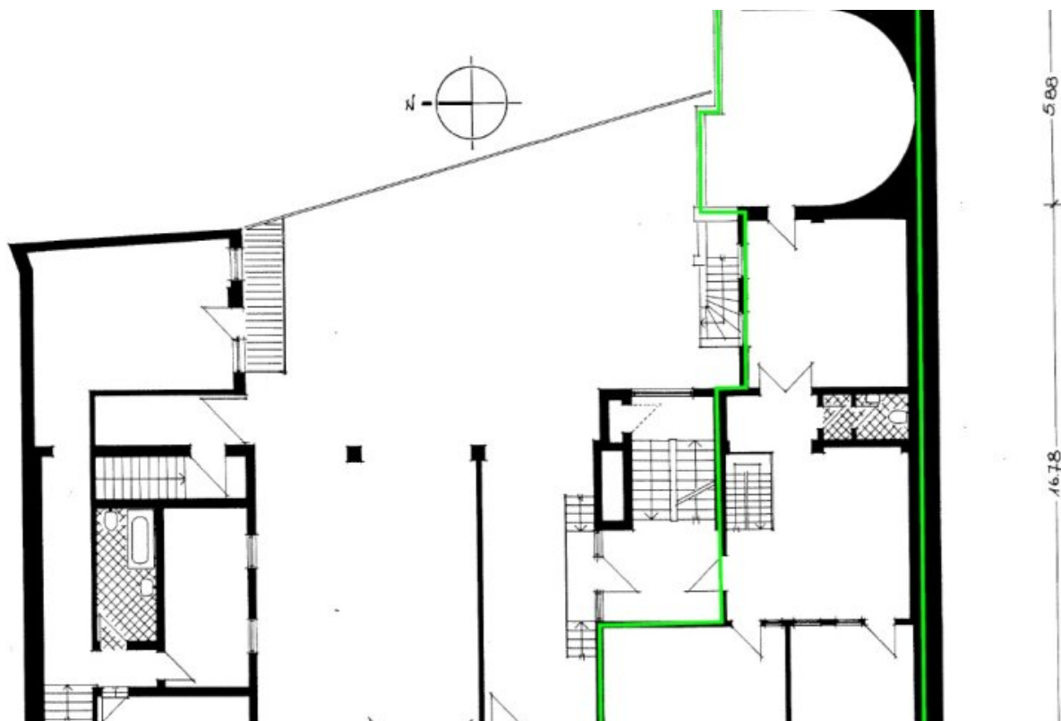
GrundrissplanEG (Grundriss)
