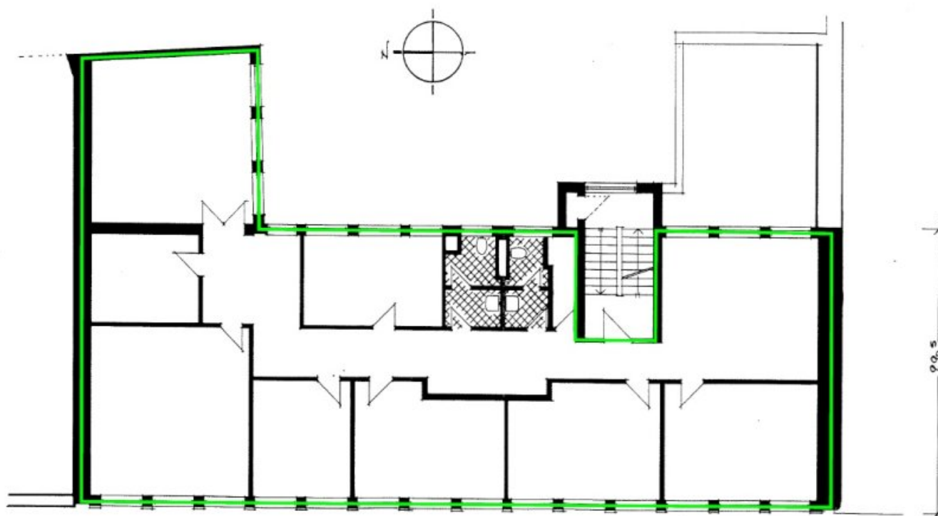
Grundrissplan1OG (Grundriss)
