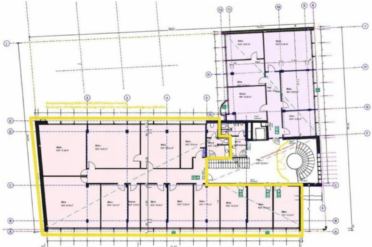
Grundrissplan3OG (Grundriss)
