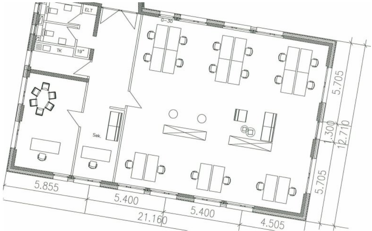
Grundrissplan (Grundriss)
