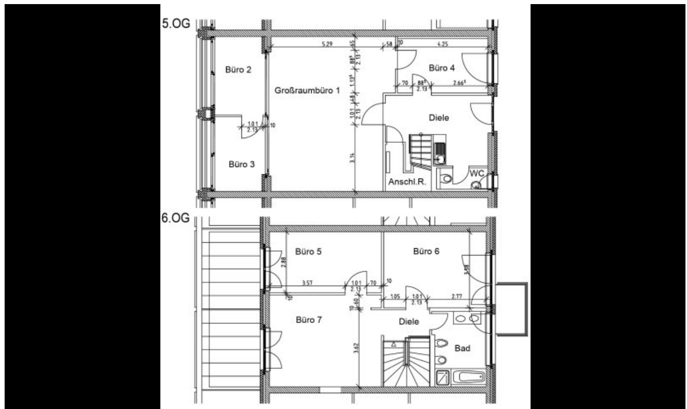
Grundrissplan 5. und 6.OG (Grundriss)
