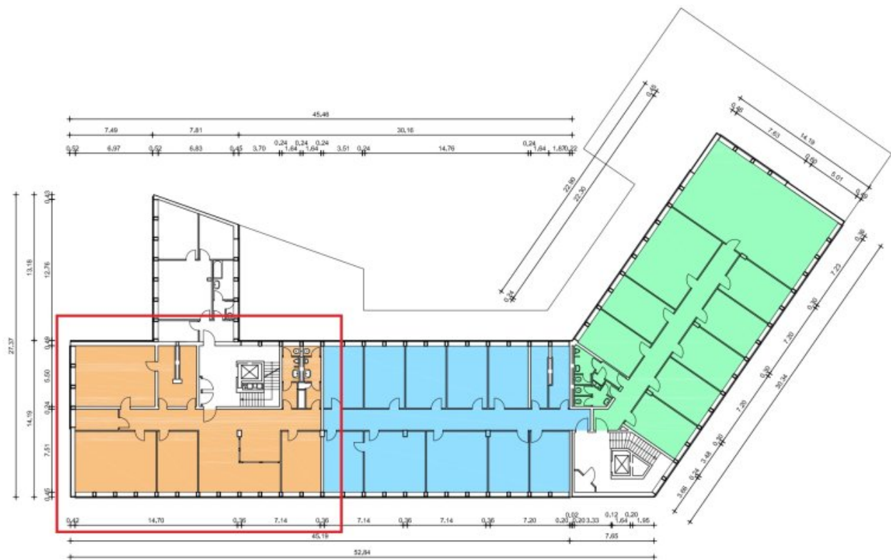
Grundrissplan 4.OG (Grundriss)
