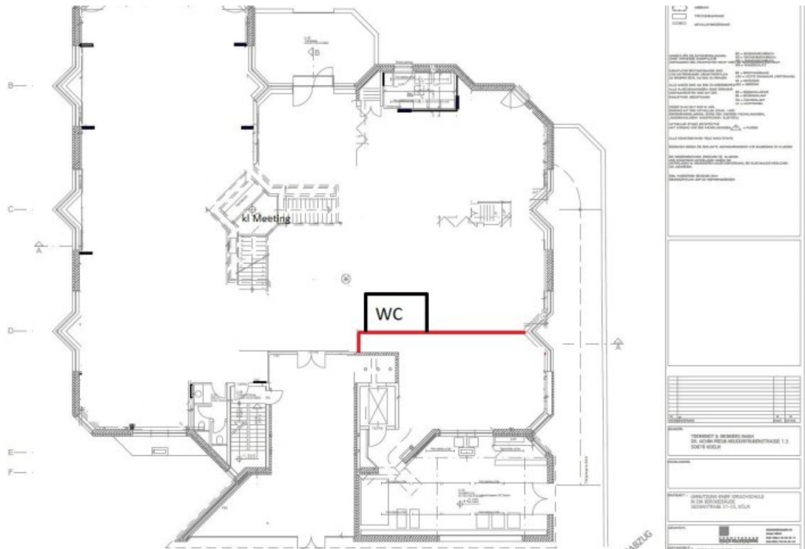
Grundriss EG (Grundriss)
