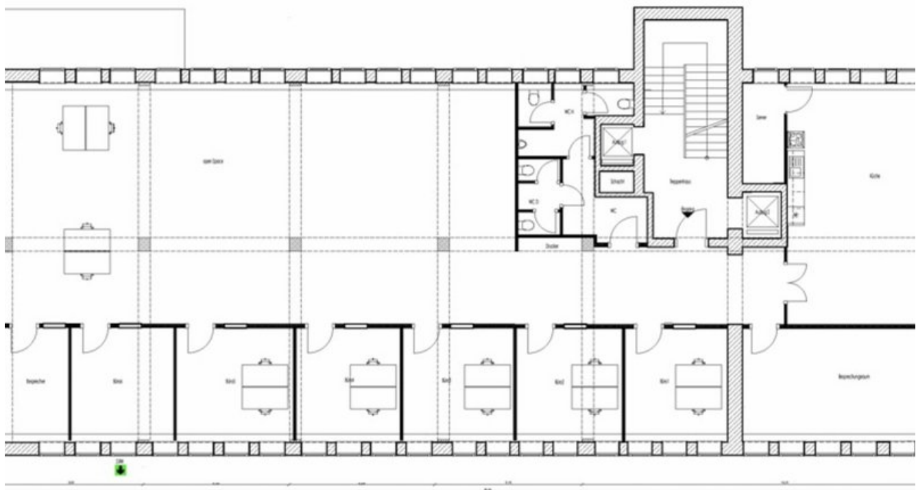
Grundrissplan 5.OG (Grundriss)
