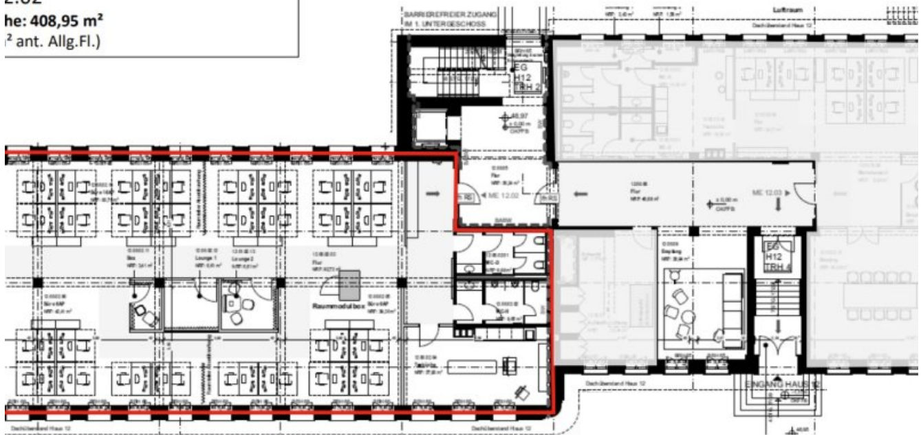
Grundrissplan CS36 (Grundriss)
