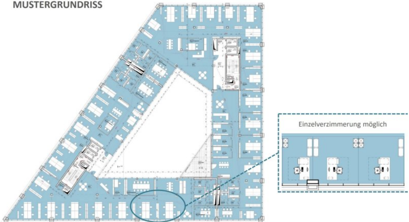
Grundrissplan (Grundriss)
