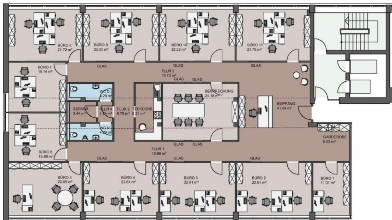
Etagengrundriss
