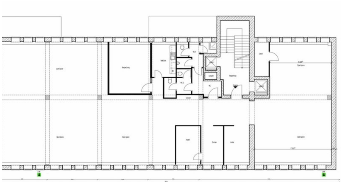
Grundrissplan 4.OG (Grundriss)
