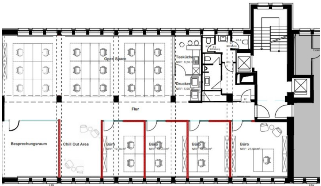
Grundrissplan2OG (Grundriss)
