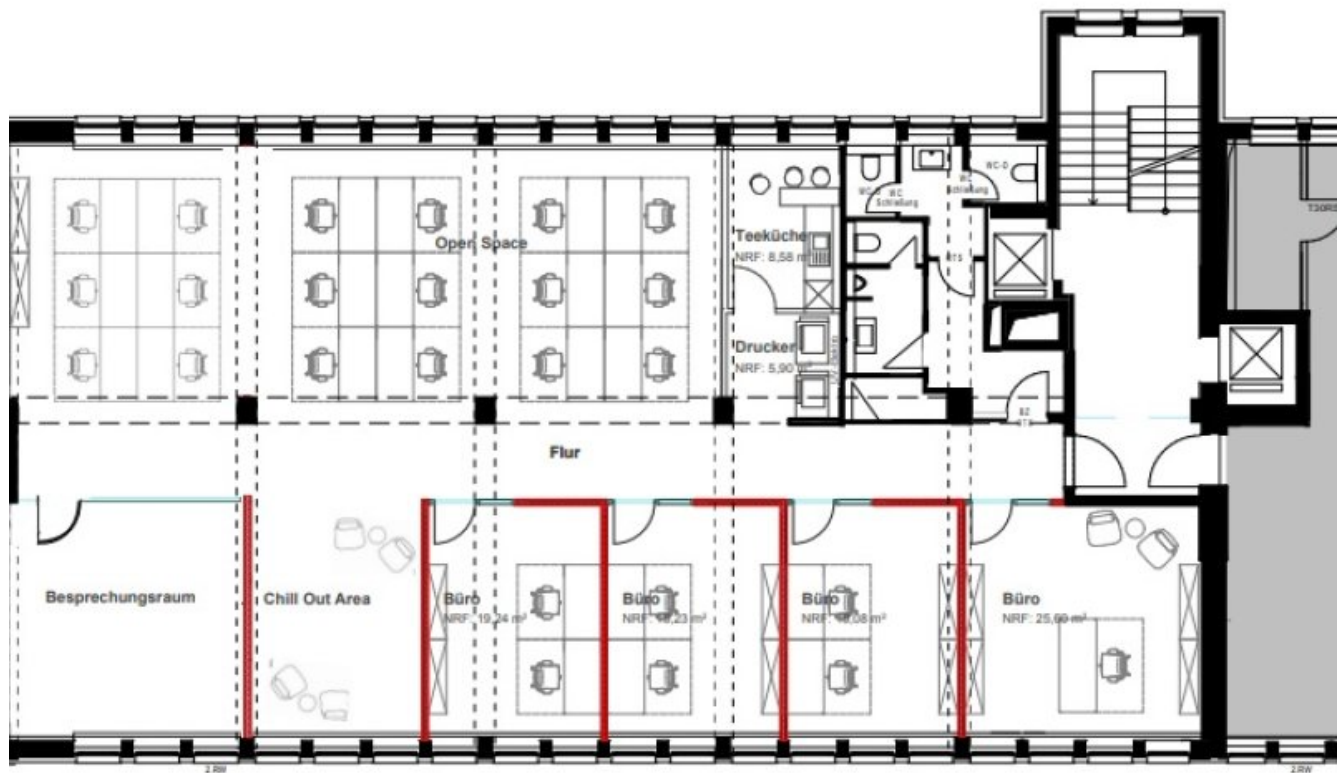
Grundrissplan2OG (Grundriss)
