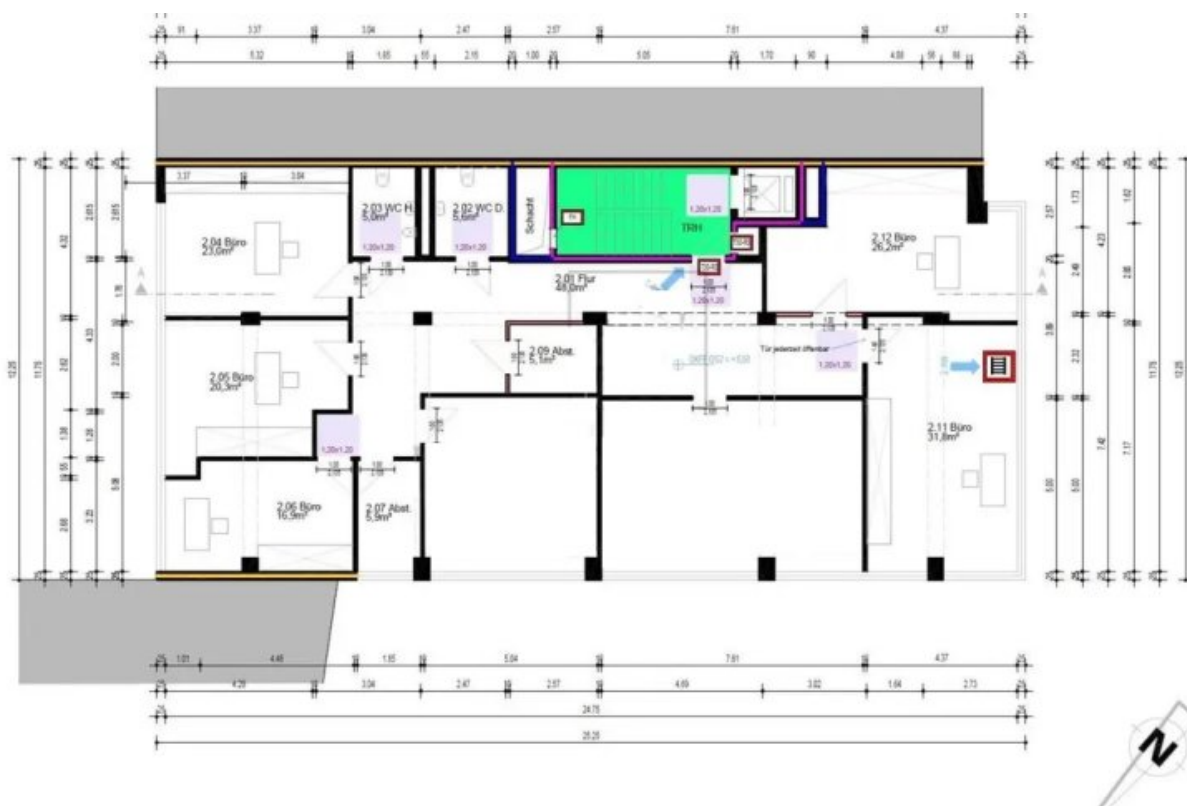
Beispielgrundriss (Grundriss)
