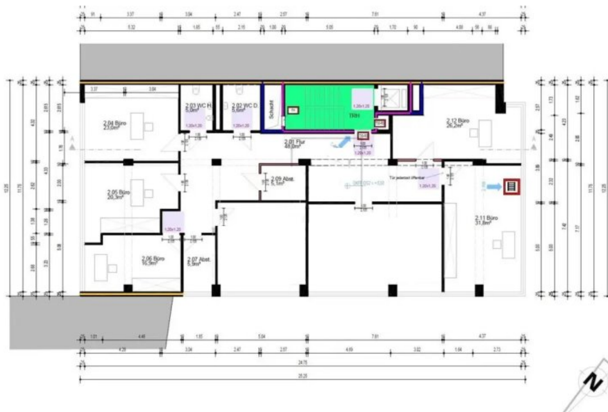
Beispielgrundriss (Grundriss)
