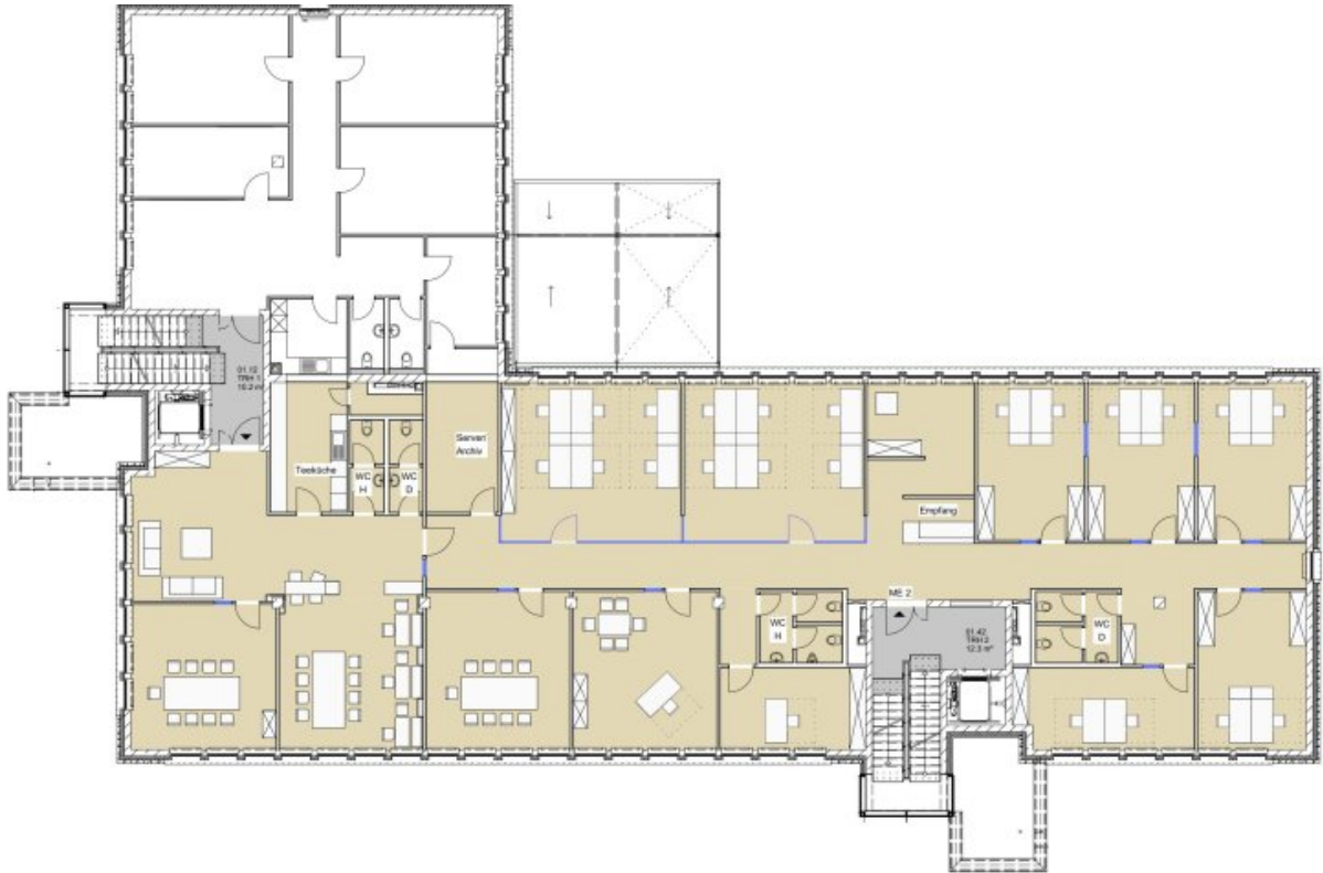
Grundrissplan 1.OG (Grundriss)
