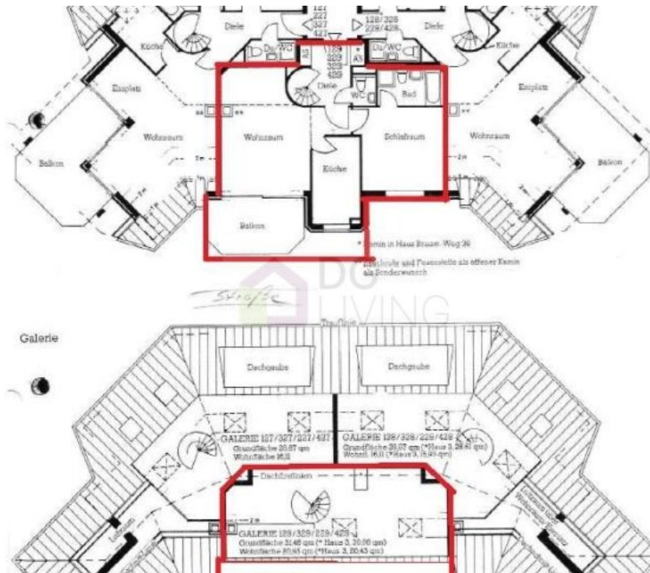
Grundrissplan (Grundriss)
