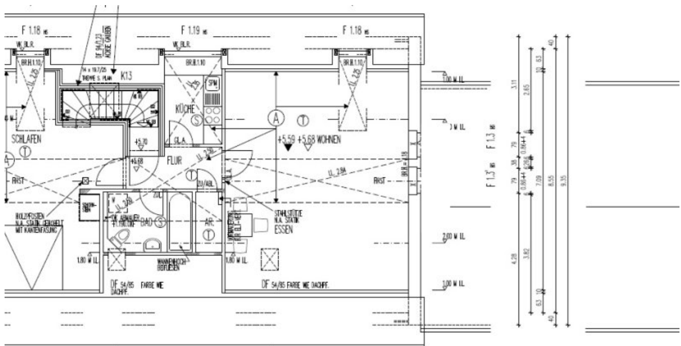
Grundrissplan1OG (Grundriss)
