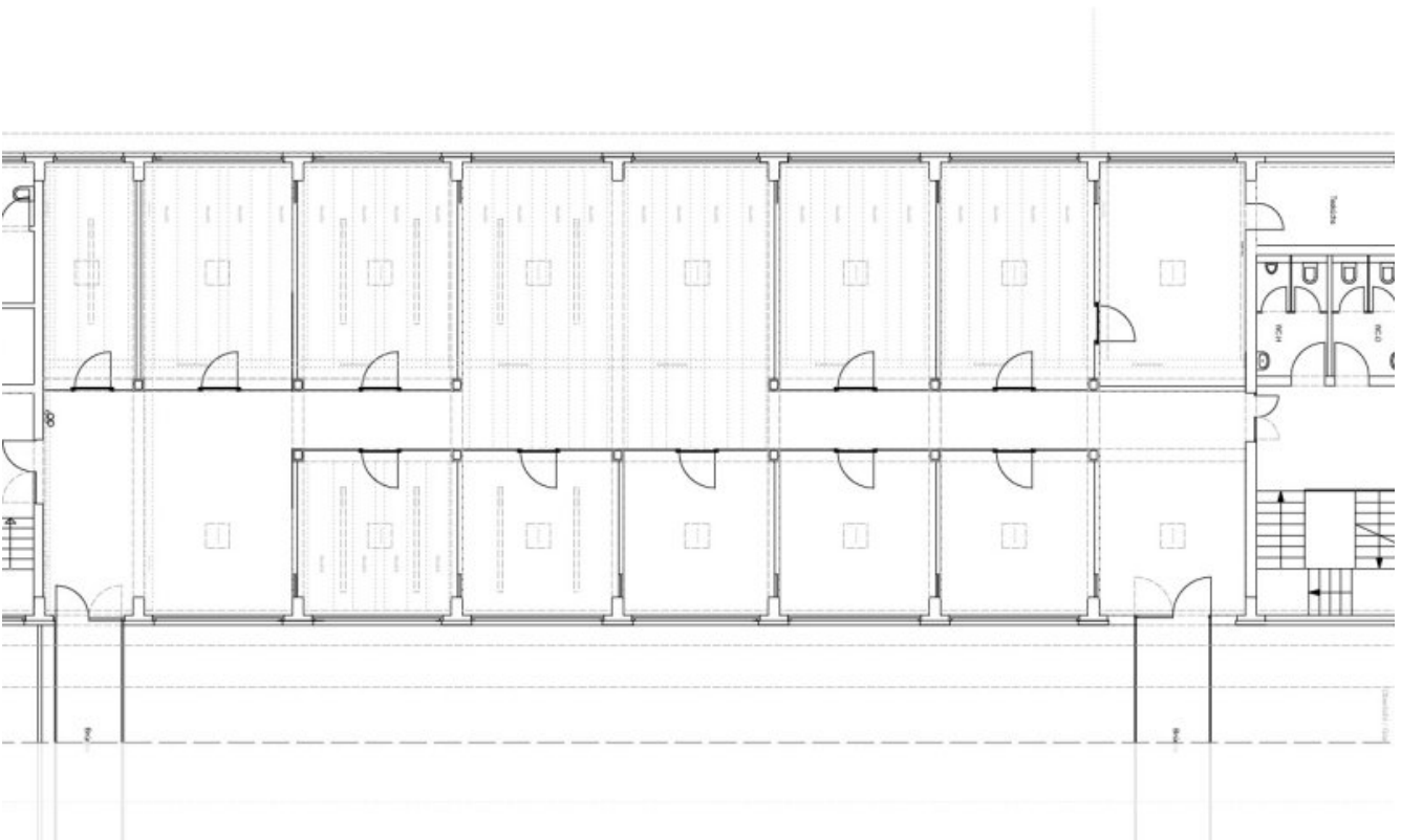
OG (Grundriss)
