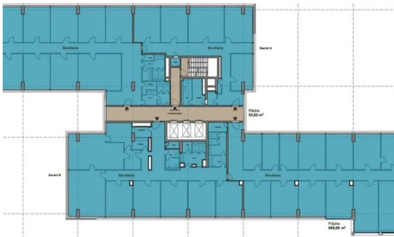
5.OG (Grundriss)
