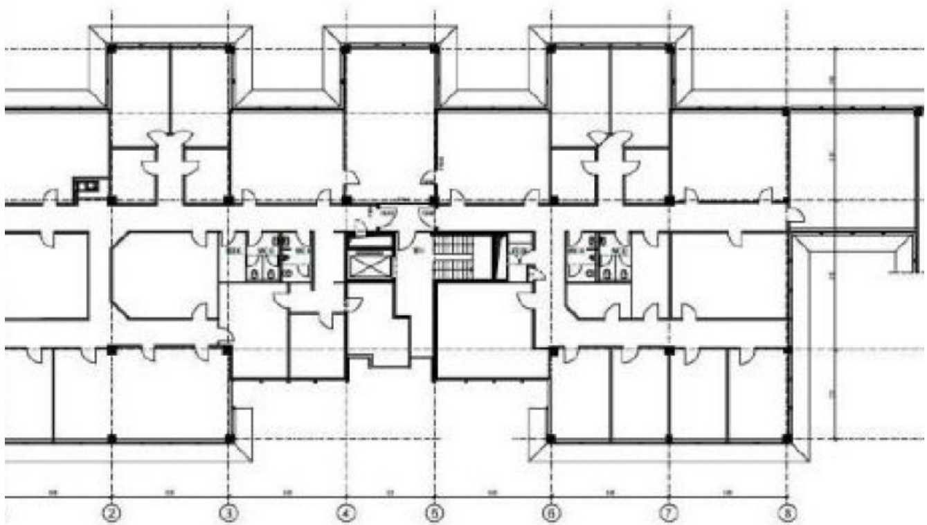
Grundrissplan (Grundriss)
