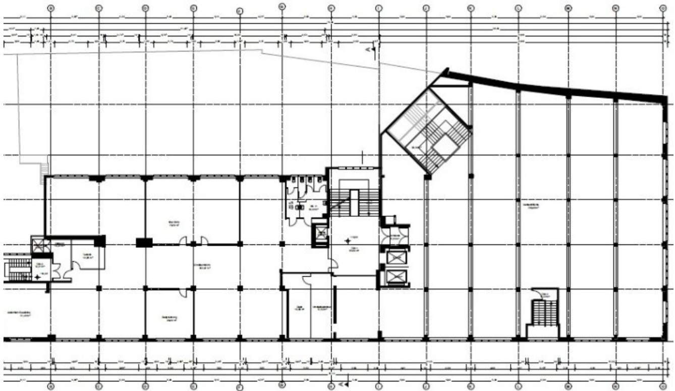
Grundrissplan 3OG (Grundriss)
