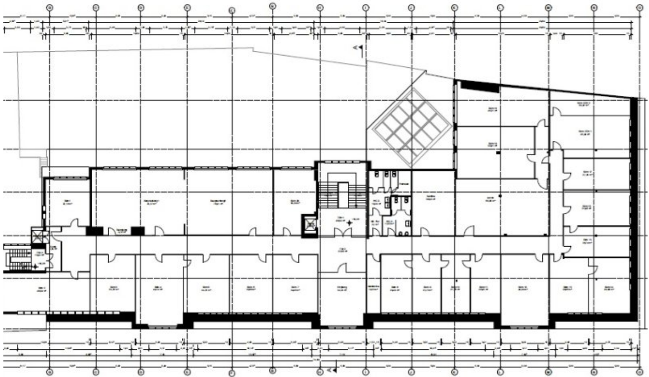
Grundrissplan5OG (Grundriss)
