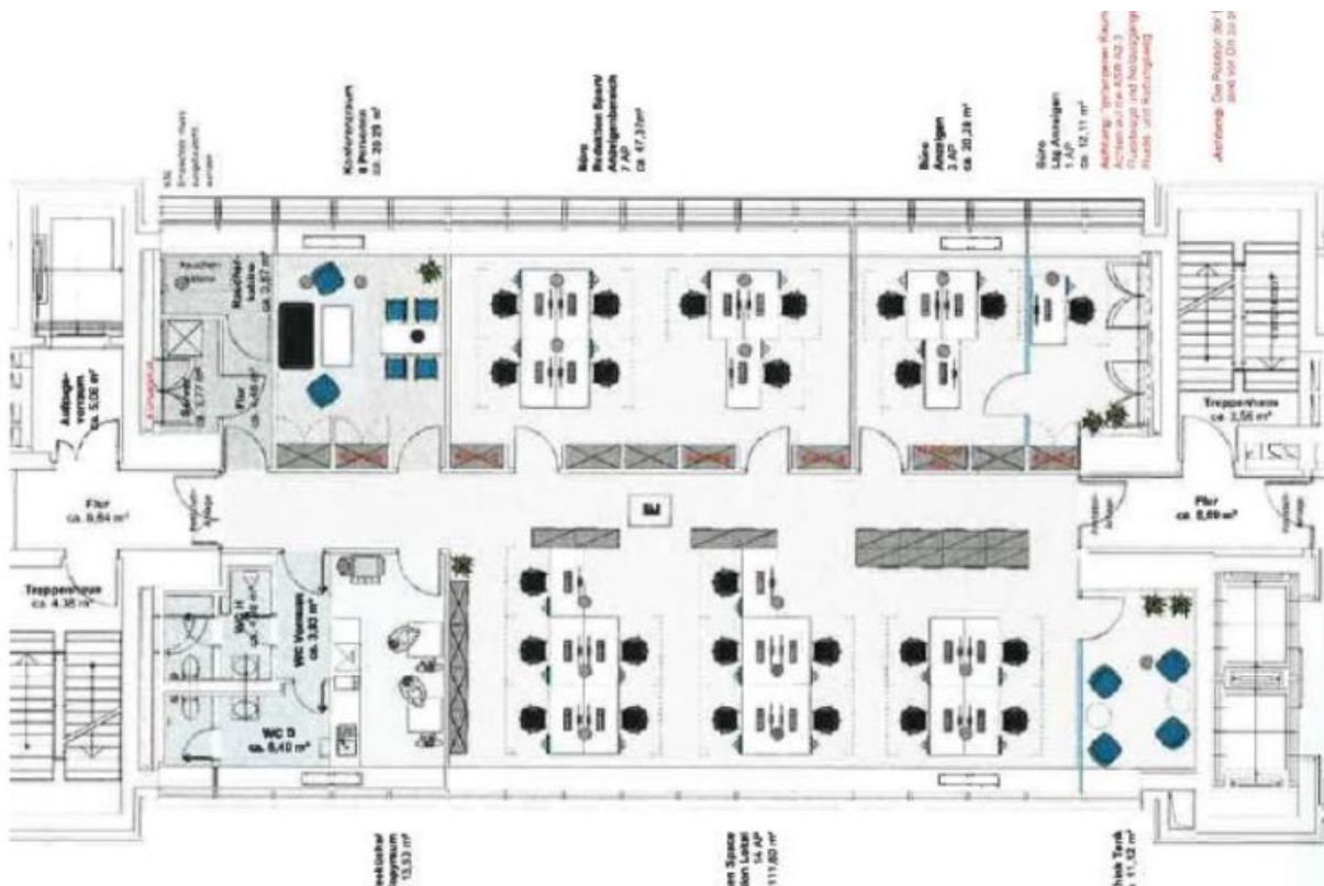
Grundrissplan50GBTE (Grundriss)
