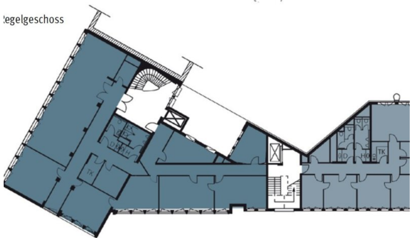
Grundrissplan (Grundriss)
