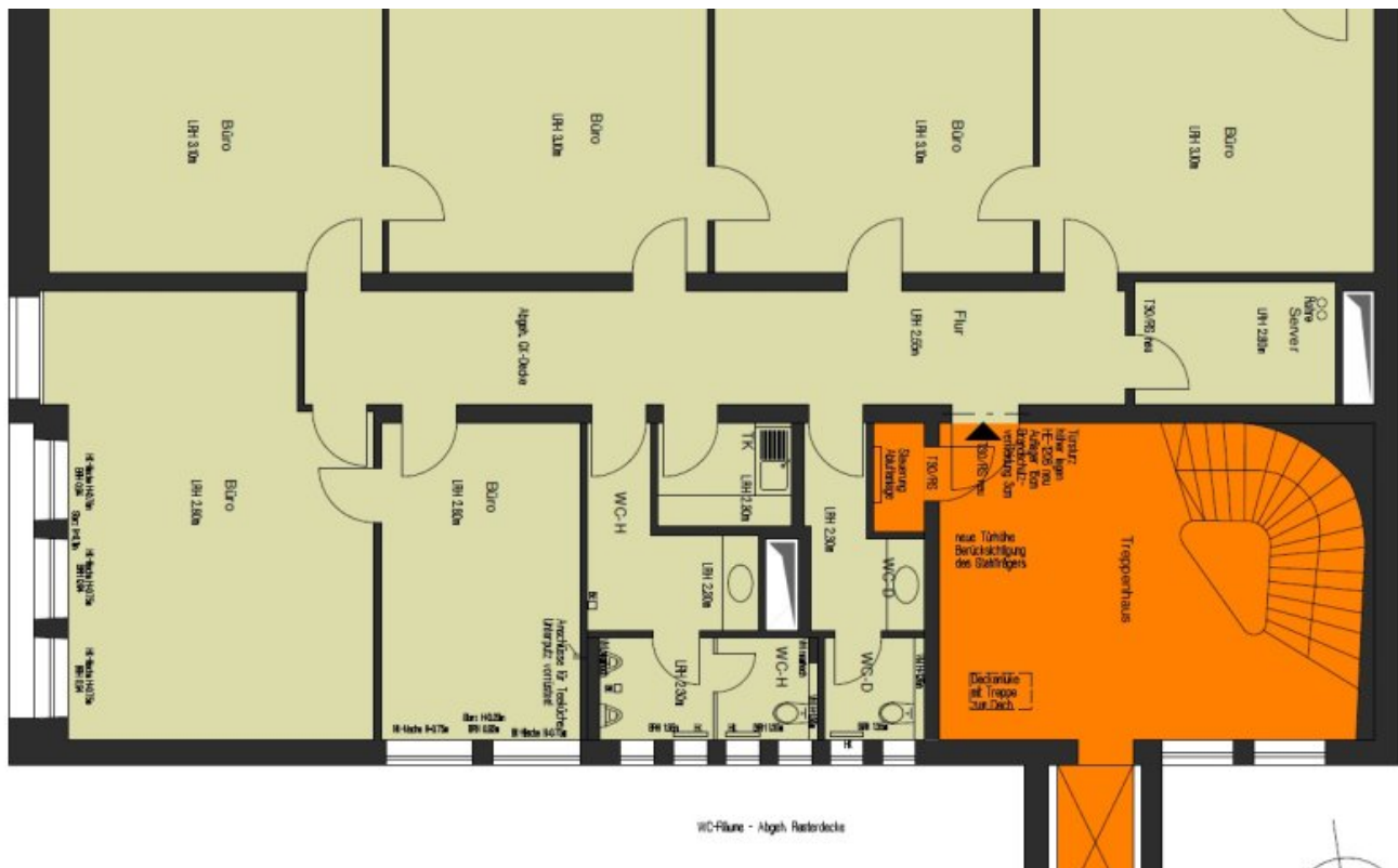
Grundrissplan 7.OG (Grundriss)
