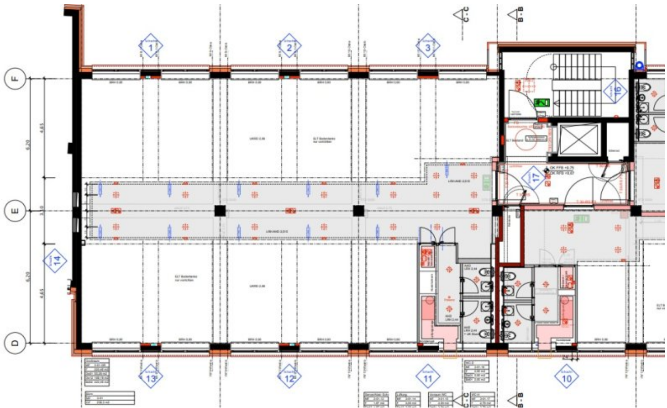
Grundrissplan 2OG Nord (Grundriss)
