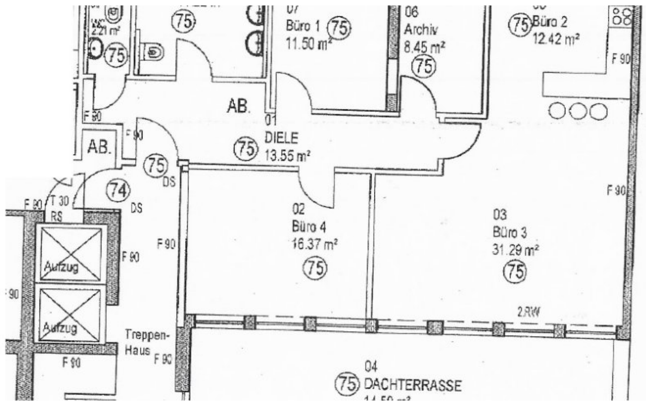
Grundrissplan 50Gre (Grundriss)
