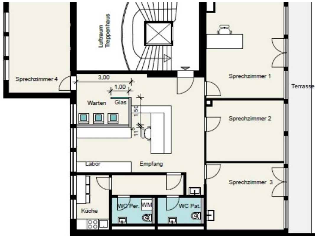
Grundrissplan (Grundriss)
