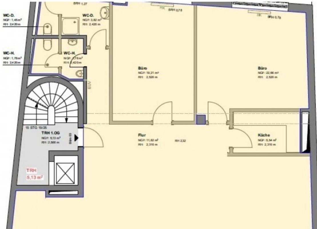
Grundrissplan (Grundriss)
